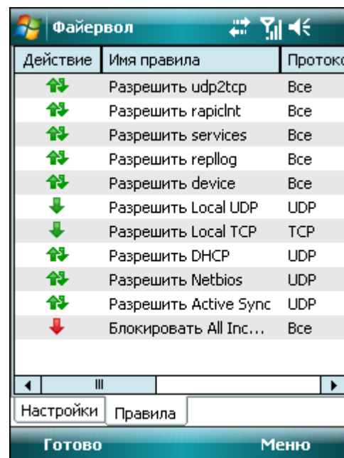
Список правил файервола
