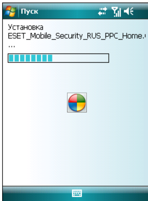
Процесс установки
