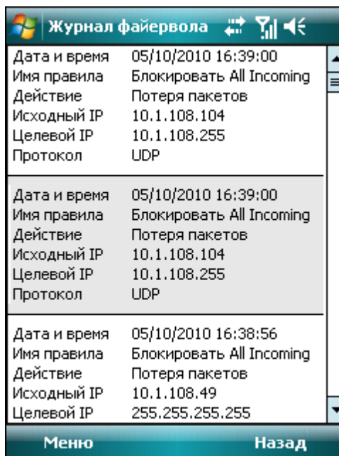
Журнал файрвола
